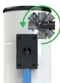
Staffa Revers con curva tecnica per intercettazione di tubo rigido aspirazione, orientata verso basso .
