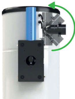
Staffa Revers con curva tecnica per intercettazione di tubo rigido aspirazione, orientata verso l'alto.
