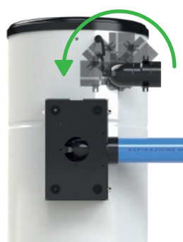
Staffa Revers con curva tecnica per intercettazione di tubo rigido aspirazione, orientata verso sx.
