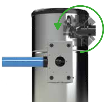
Staffa Revers con curva tecnica per intercettazione di tubo rigido aspirazione, orientata verso dx .
